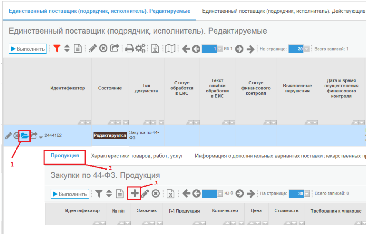
Рисунок 8 - Добавление продукции
